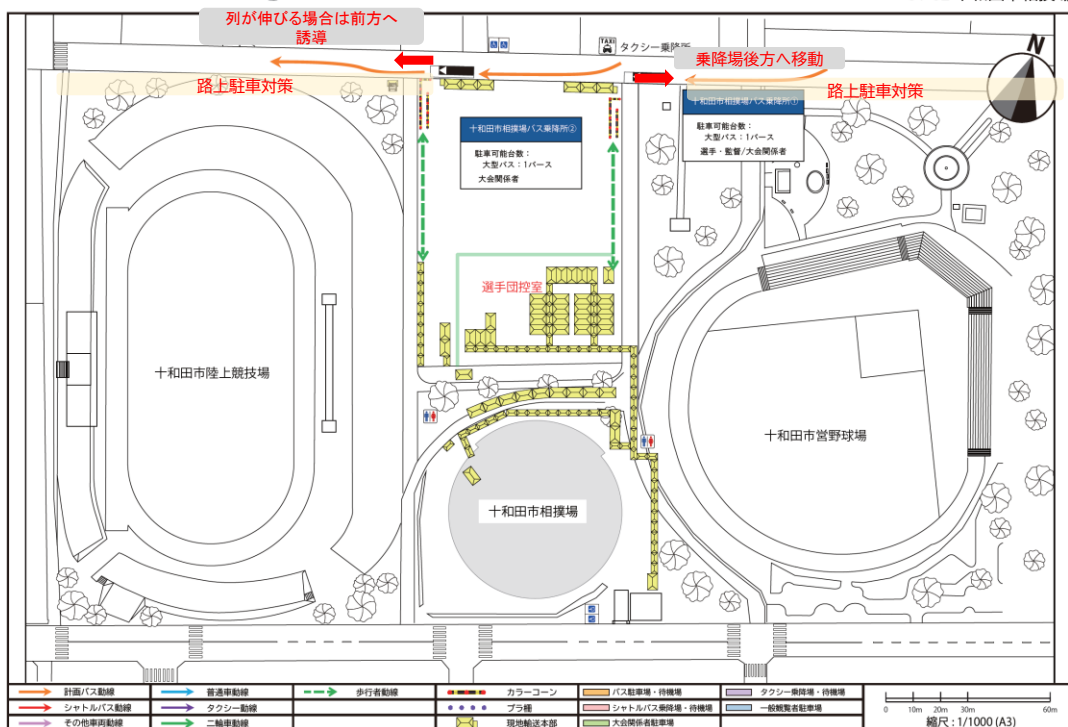
【十】 駐車場利用計画 01-02 十和田市相撲場
