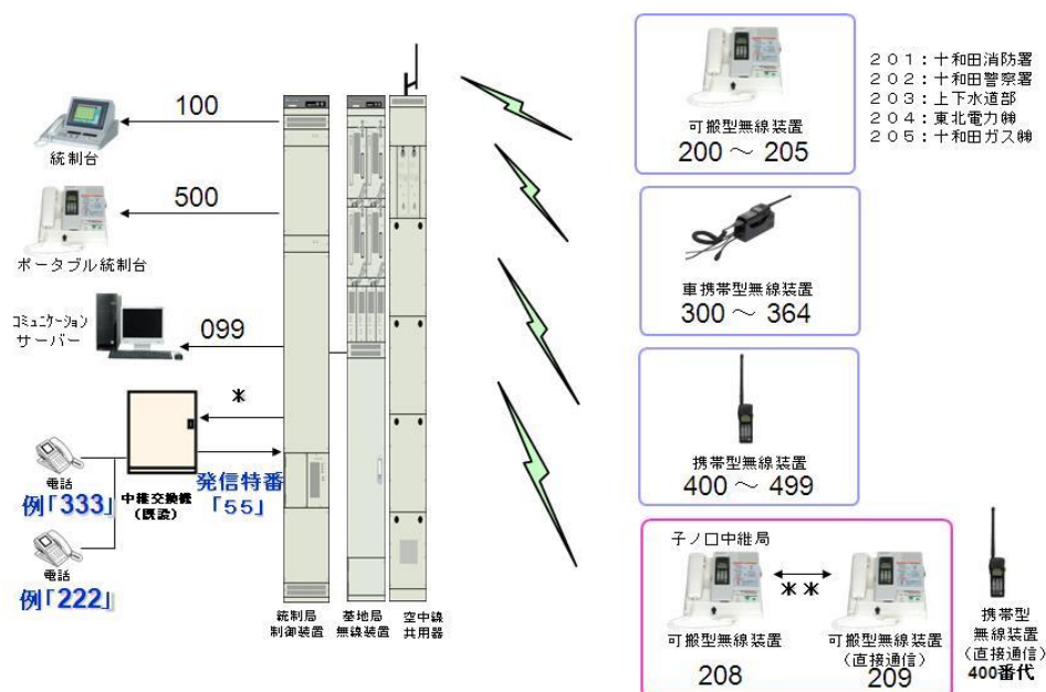
移動系防災行政無線系統図
