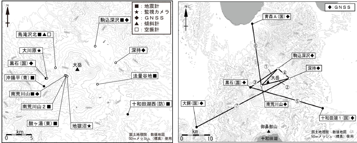
八甲田火山観測点配置図
