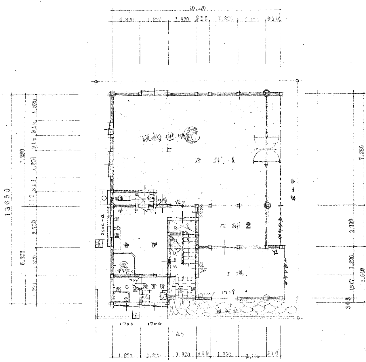
1F 平面図 S1/100
