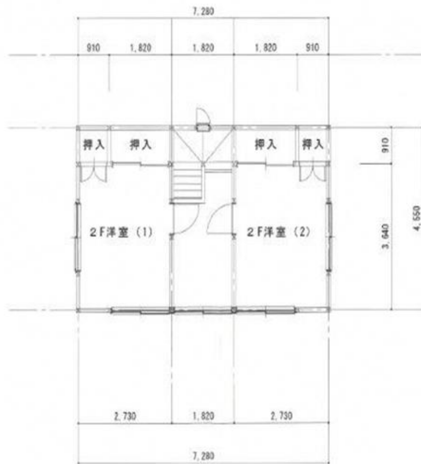
2階平面図
