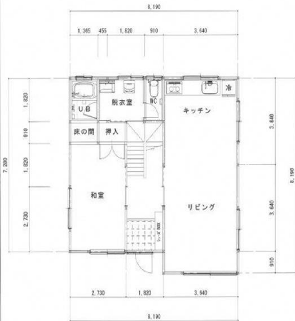
1階平面図
