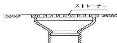
図 1－1 4 ストレーナーの例（目皿）
