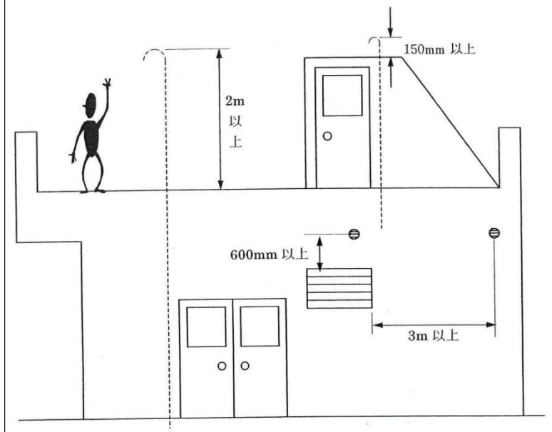
図 1 - 3 6 通気管の開口位置
