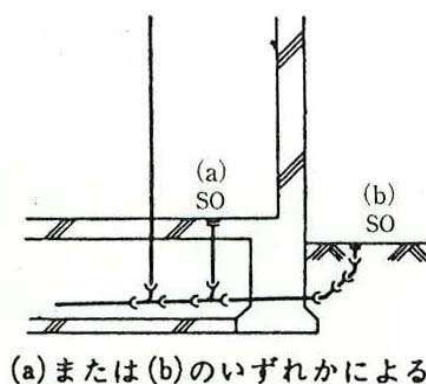
図1-15 掃除口の取付け状態の例
