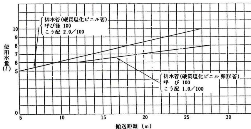
図 1 - 2 2 使用水量による搬送距離
