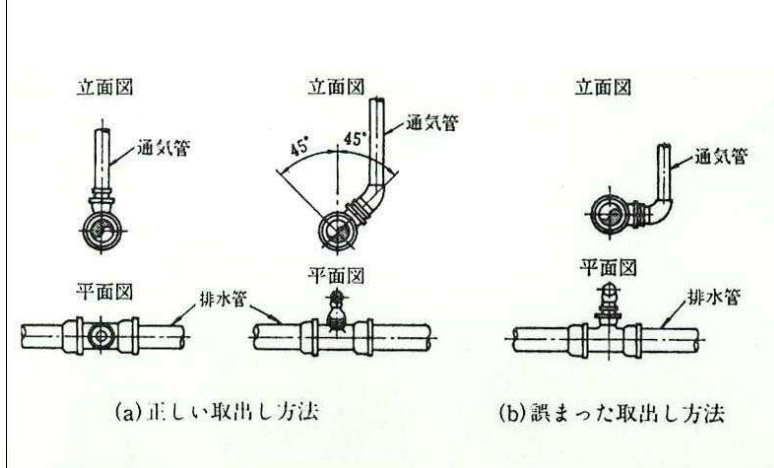
図 1 - 3 7 通気管の取出し方法
