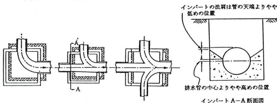
図2-7 排水管が屈曲している場合のインバート築造
