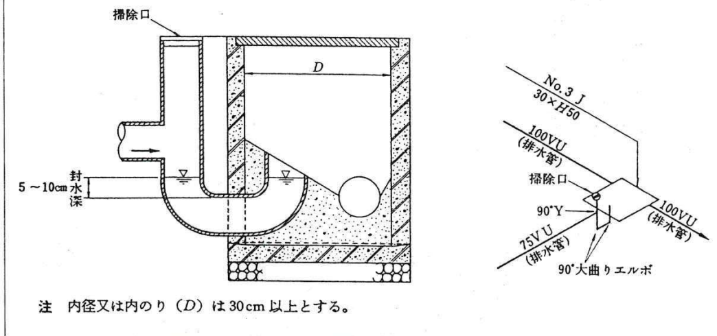
図 1-43 J型トラップますの例
