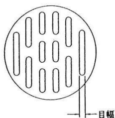
図 1－1 4 ストレーナーの例（目皿）
