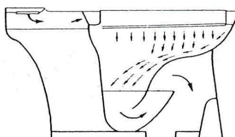
図 1-17 洗落し式
