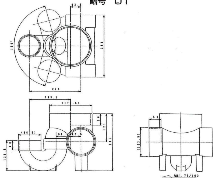
図 1 - 5 2 トラップインバートますの例 その 1 (中間点) 略号 UT
