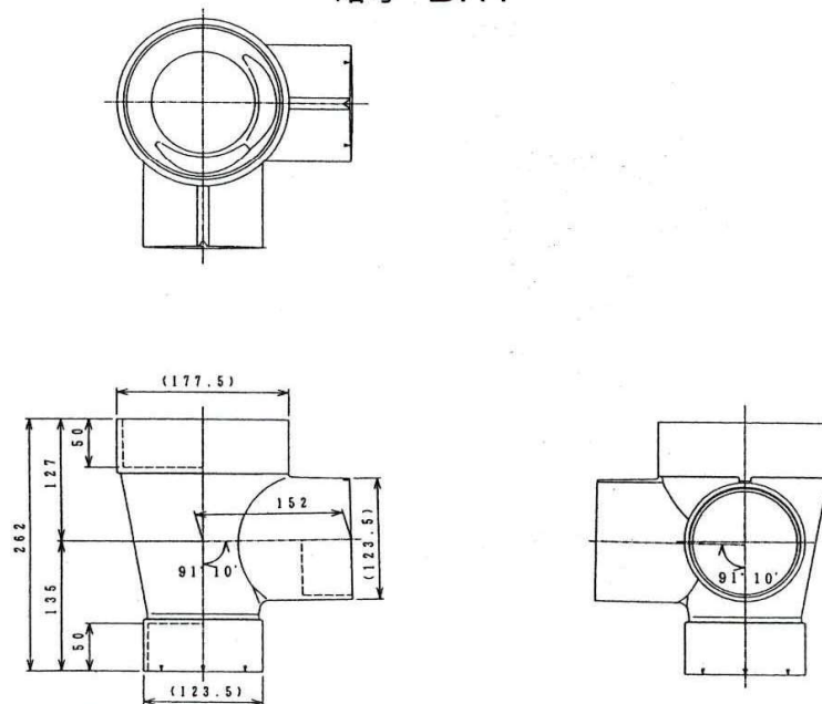
図 1-56 ドロップインバートますの例 その2 略号 DRY
