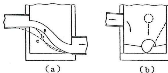
図2-8 上・下流の排水管に相当の落差がある場合のインバート築造
