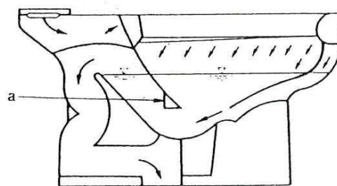
図 1-19 サイホンゼット式
