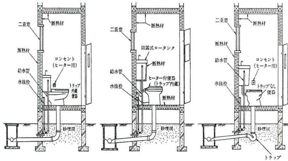
図 1 - 2 5 寒冷地の水洗便所の例
