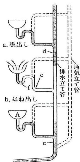
図1-11 はね出し作用
