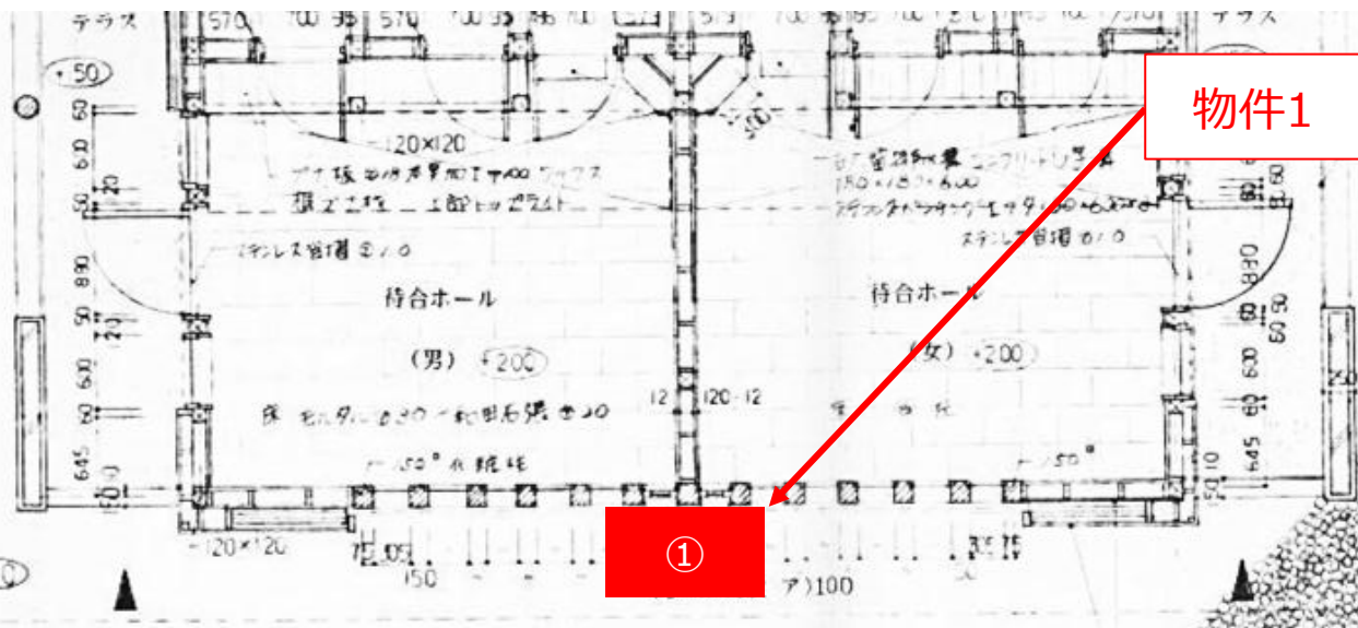
十和田市宮宇樽部キャンプ場 シャワー棟(軒下) 設置個所平面図
