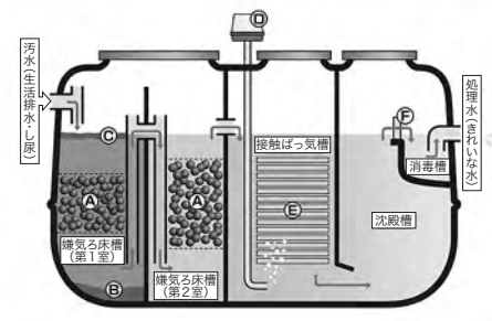
合併処理浄化槽
