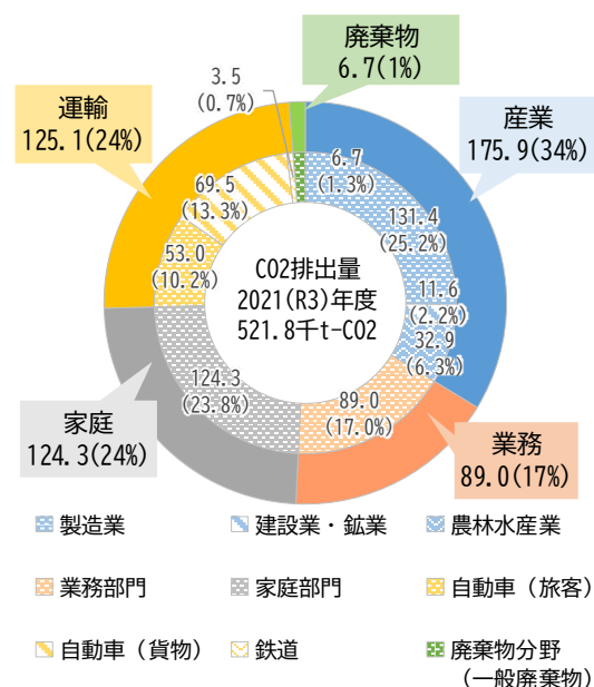
図 3-2 2021 年度の C02 排出量 部門分野別内訳
