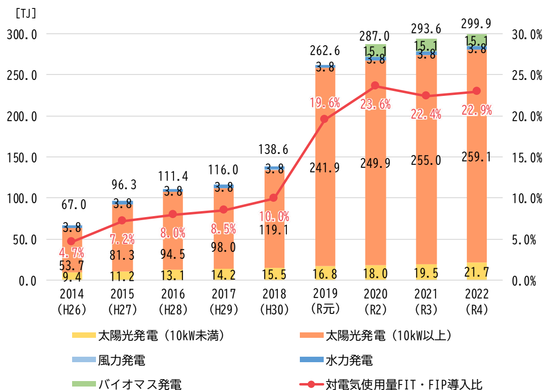
図 2-33 再エネ発電量（FIT）の推移
