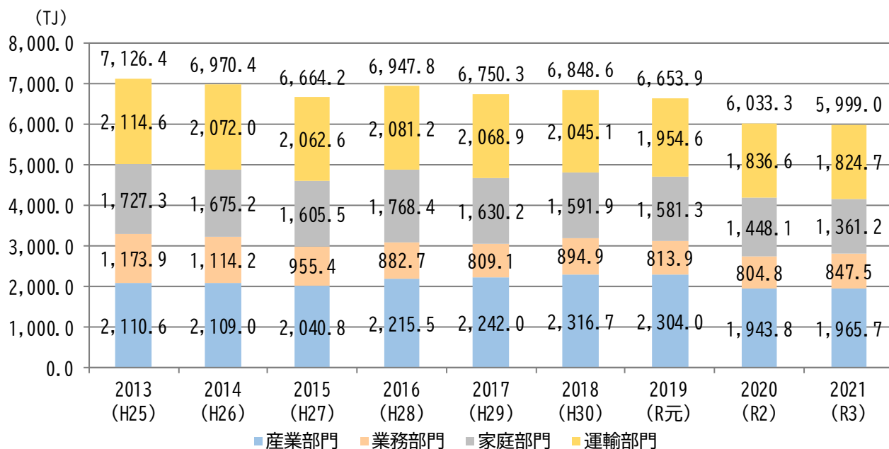
図 2-28 2013-2021年度のエネルギー消費量の推移
