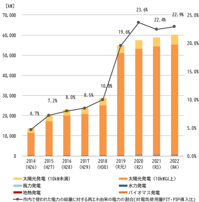
図 2-31 再生可能エネルギーの導入設備容量の推移
