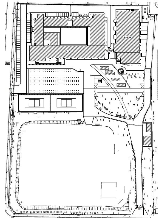
三本木中学校 配置図
