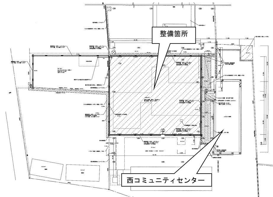
十和田湖支所跡地整備 平面図（案）
