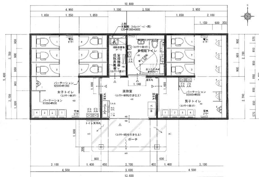
奥入瀬溪流館駐車場トイレ平面図（案）
