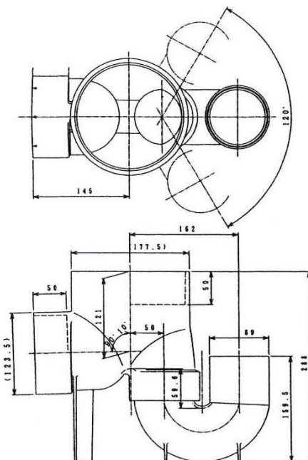
図 1-54 トラップインバートますの例 その3
