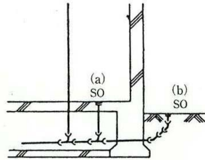
図1-15 掃除口の取付け状態の例
