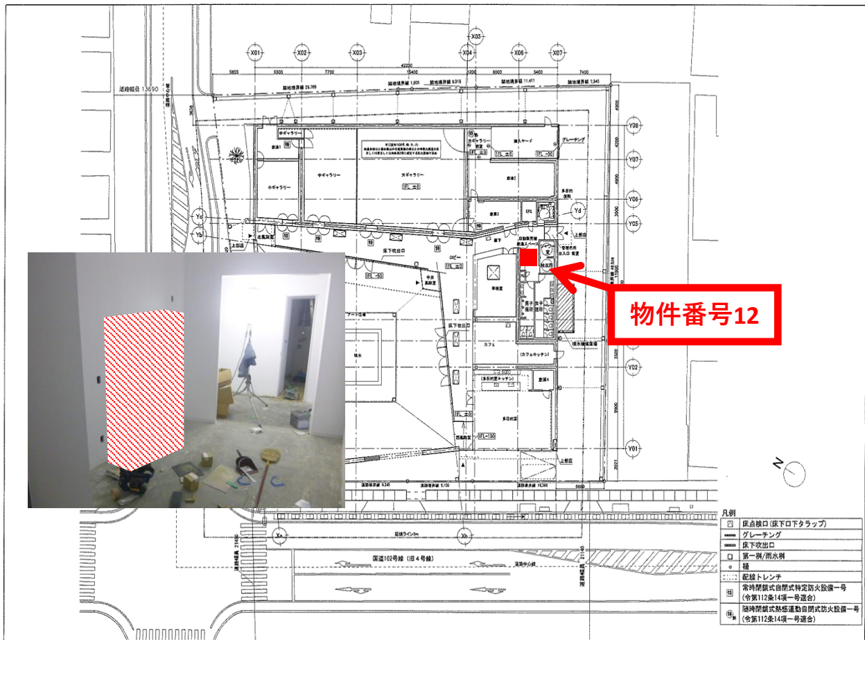
十和田市地域交流センター 自動販売機設置箇所平面図 (配置図)
