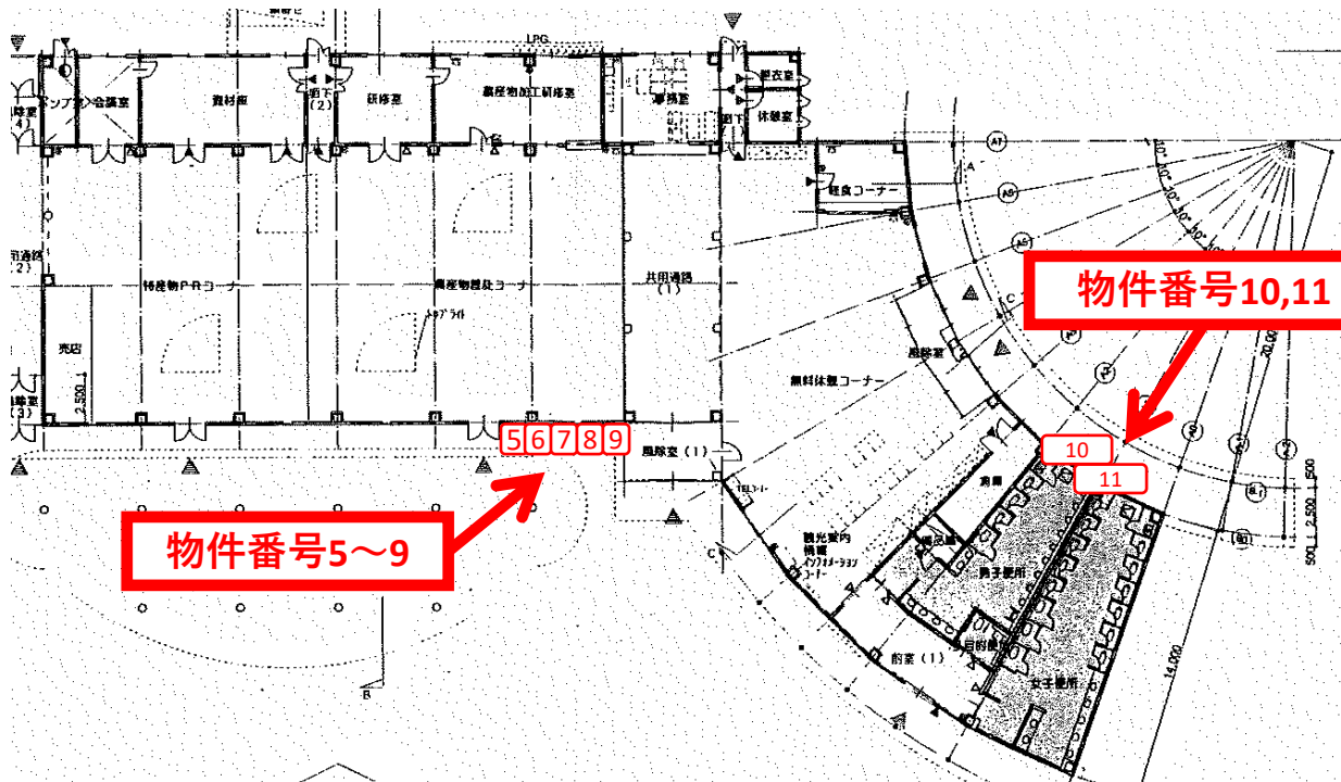
道の駅とわだ 自動販売機設置箇所平面図 (配置図)
