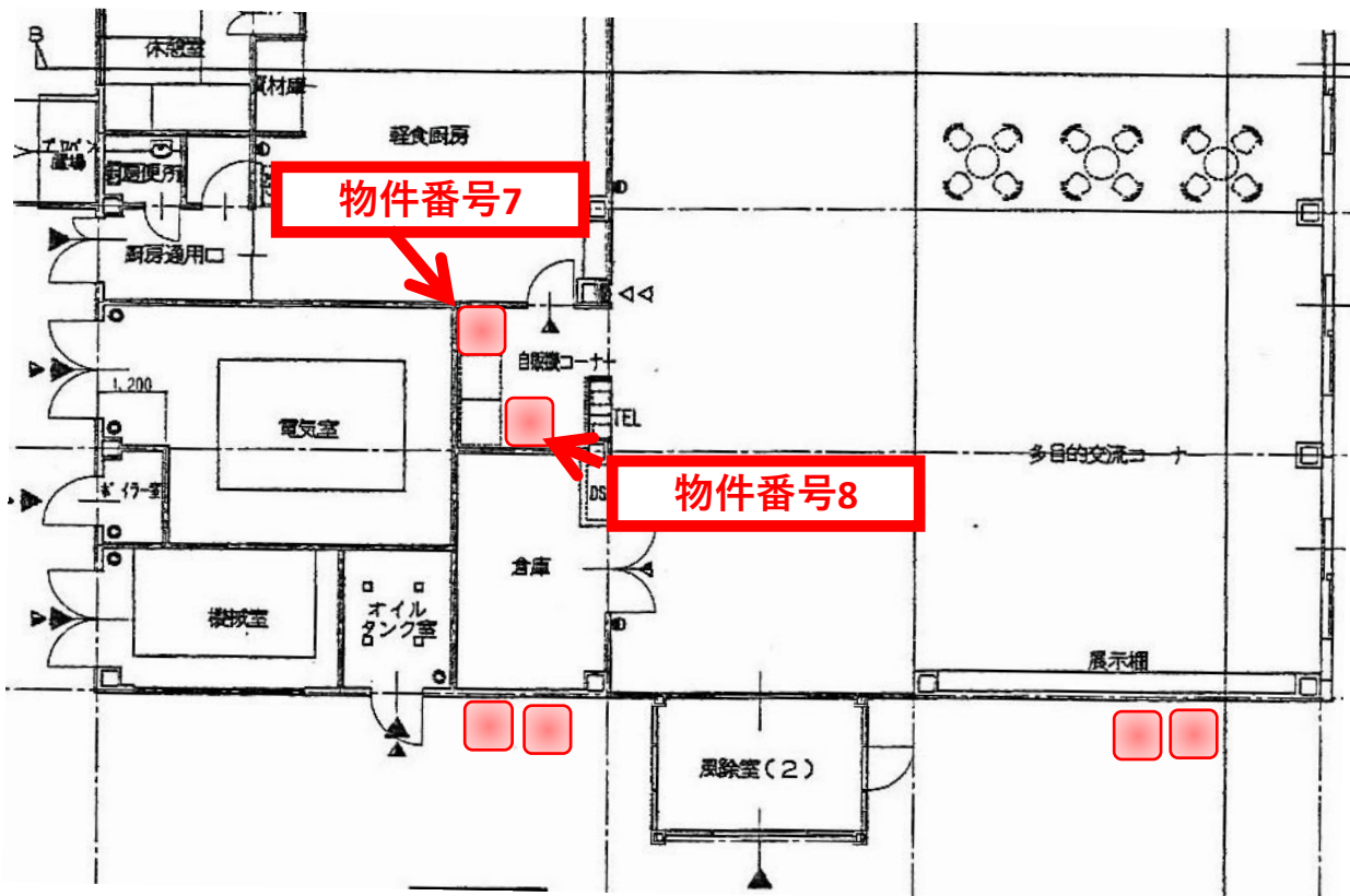
馬事公苑交流館 自動販売機設置箇所平面図（配置図）
