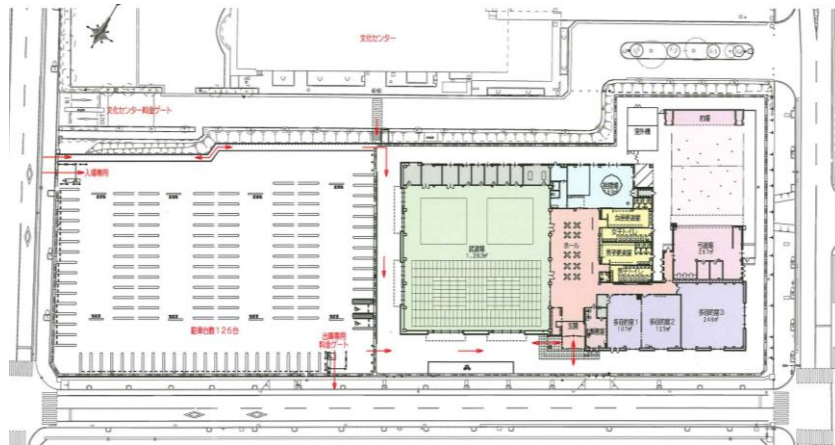
(新) 志道館平面図
